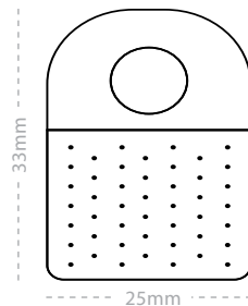
HOLE TAB
