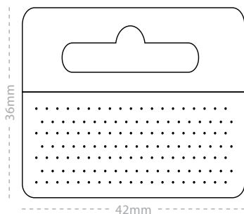
EURO TAB
